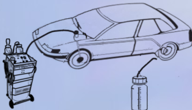
Dispositivo di manutenzione del freno collegato all'autovettura
